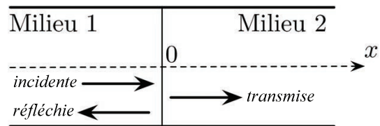
FIGURE 5 – Dioptre acoustique.
