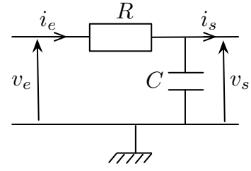
FIGURE 4 – Filtre.
